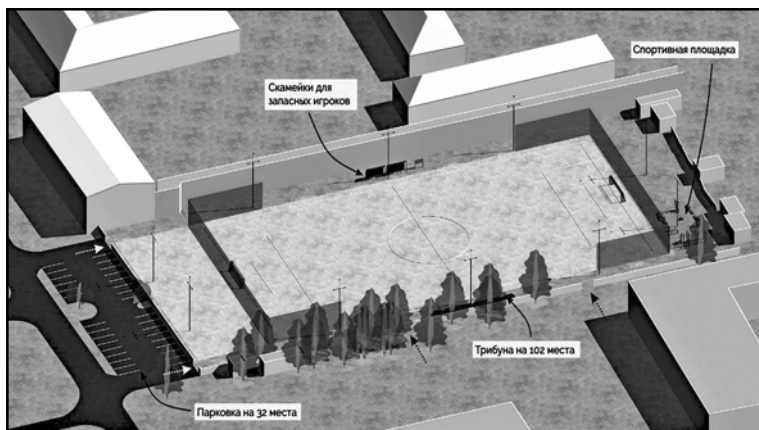
Дизайн-проект «Стадион МКУ «ГМЦ», ул. Кирова, 41»
