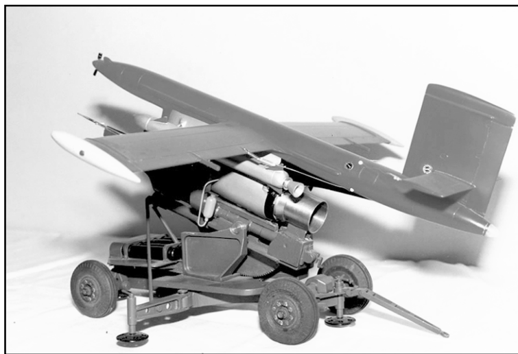
Один из первых отечественных БПЛА – разведывательный Ла-17Р
