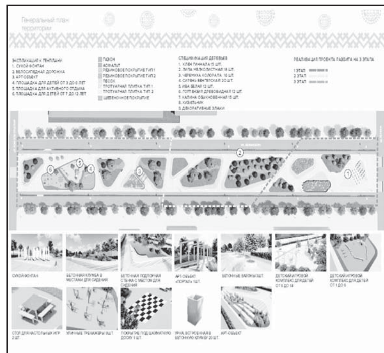
Генеральный план благоустройства аллеи по ул. Белинского
